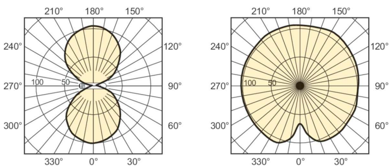
LDL_SONTHORT_0001-Light distribution diagram
